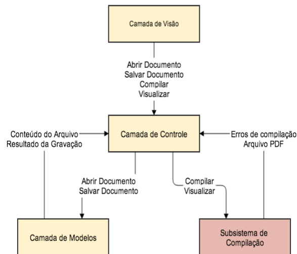
Figura 12: Arquitetura do IFBATEX
