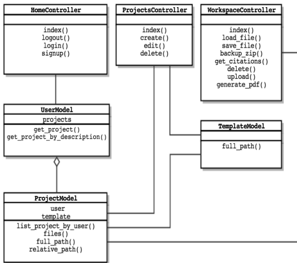
Figura 13: Diagrama de classes
