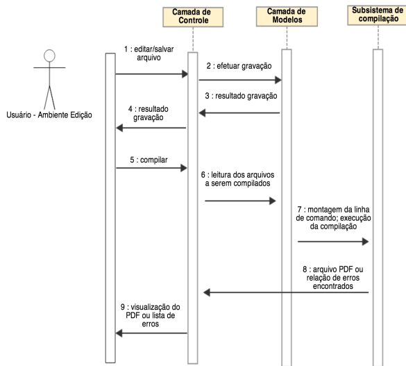
Figura 14: Diagrama de seqüência
