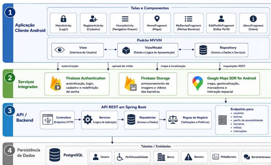
Figura 4 - Visão arquitetural do sistema
